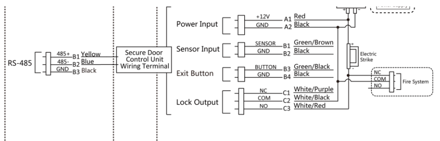
Рисунок 4- 8 Подключение устройства
