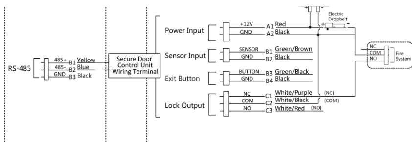
Рисунок 4-6 Подключение устройства
