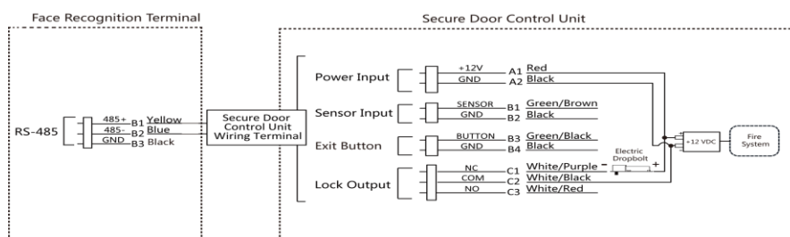
Рисунок 4-4 Подключение устройства
